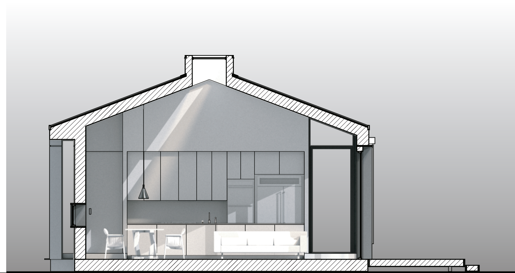
Section A: Living Room
